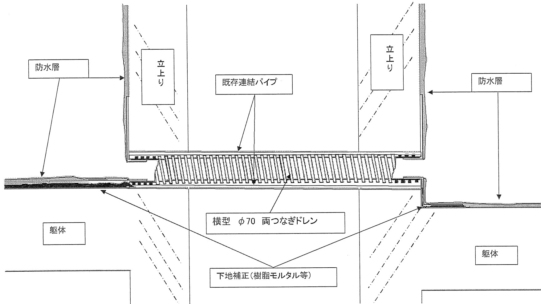
別棟一括排水連結パイプ経年劣化部分の補修
